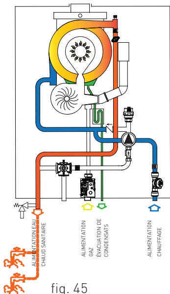
MODE TIRAGE (RECIRCULATION PAS ACTIVÉE)
