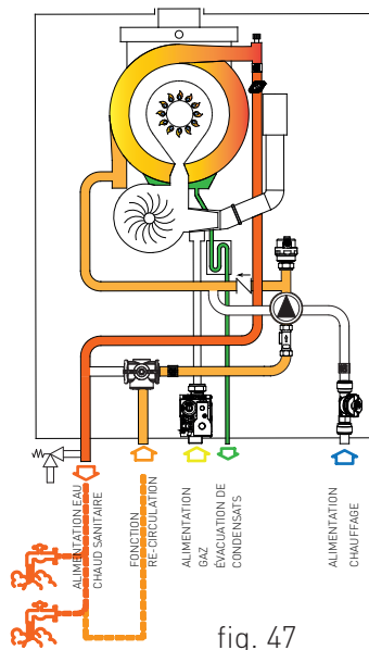
MODE RECIRCULATION (APRÈS-CIRCULATION ACTIVÉE)
