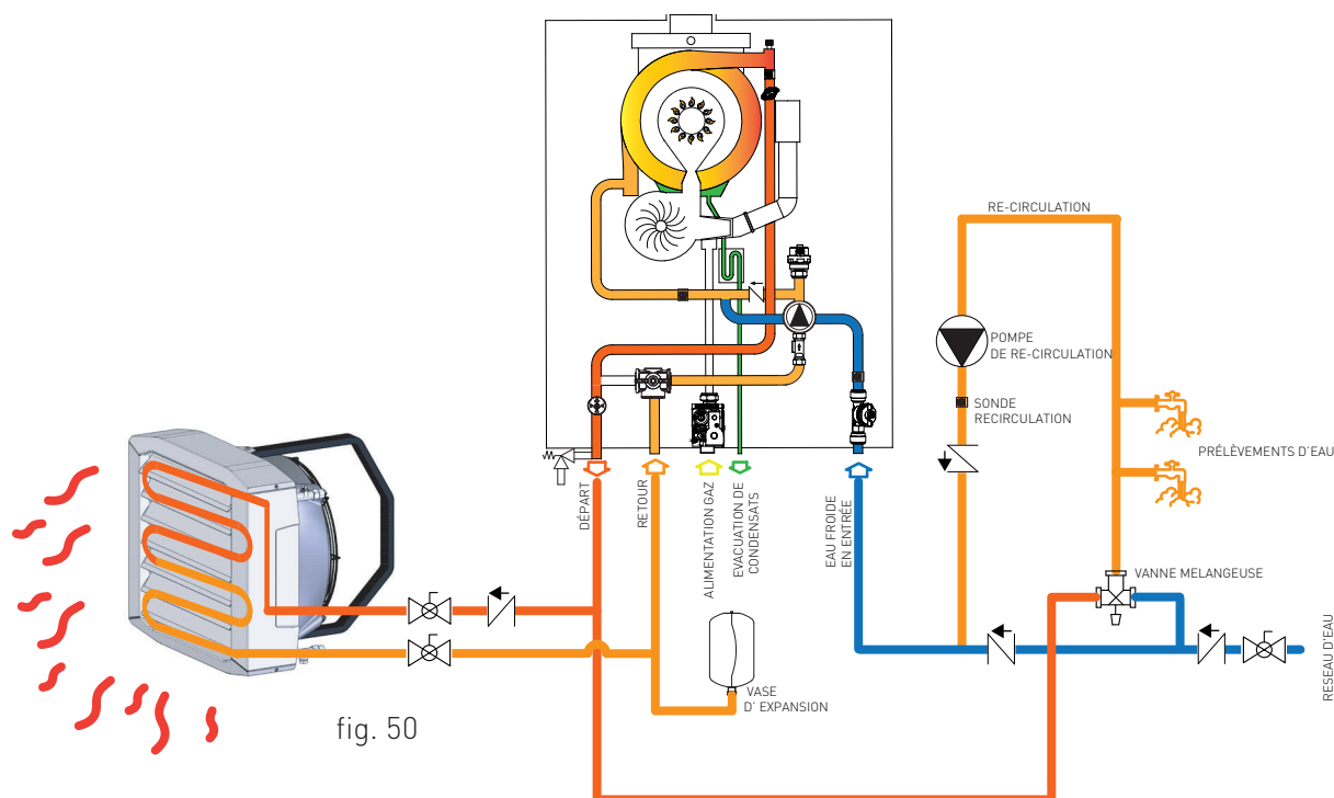
MODE MIXTE (ECS + CHAUFFAGE) AVEC RECIRCULATION EXTERNE
