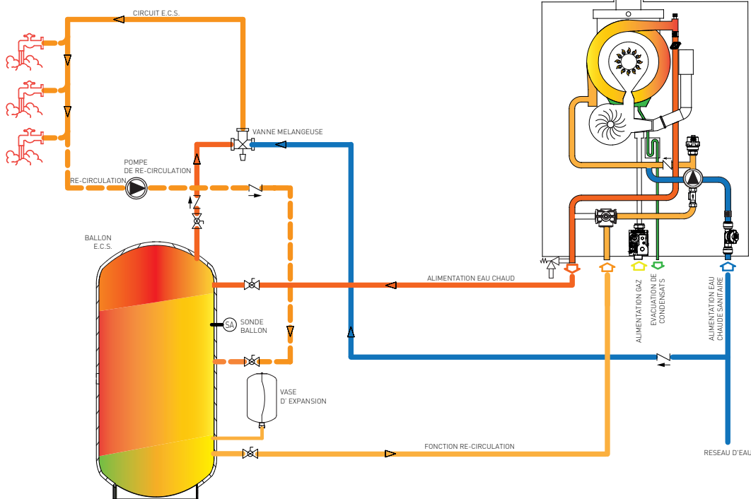
PRODUCTION D'E.C.S. PAR L'AIDE D'UNE CUVE
