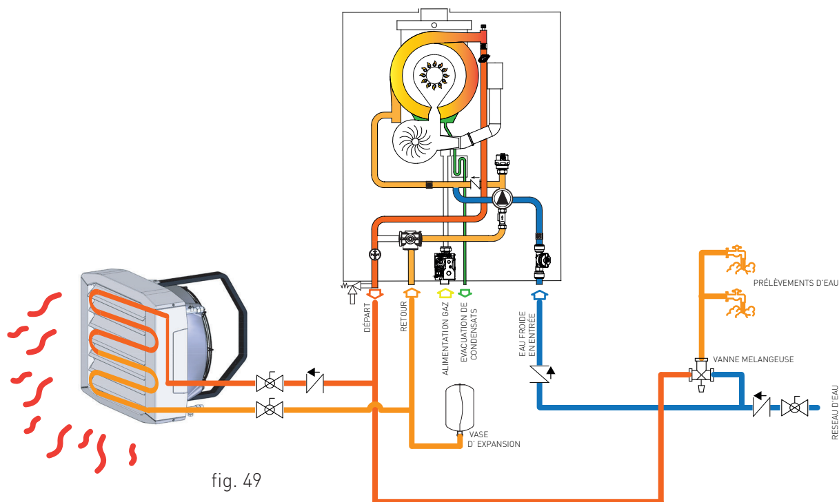
MODE MIXTE (ECS + CHAUFFAGE)
